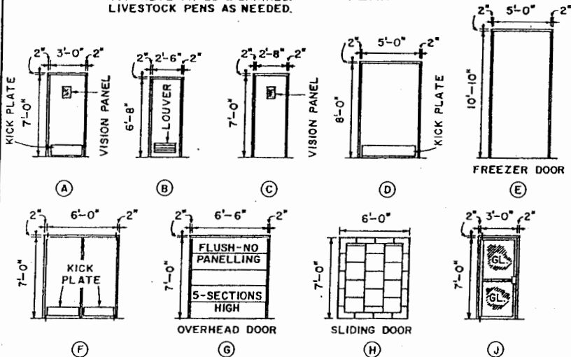
DOOR SCHEDULE
