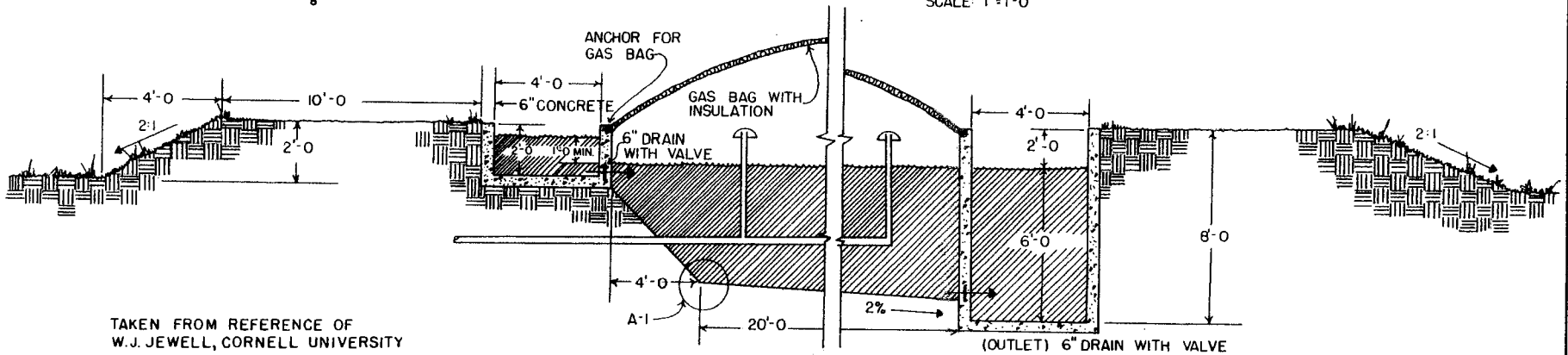
END SECTION SCALE: \frac{3}{8} " = 1'-0"
