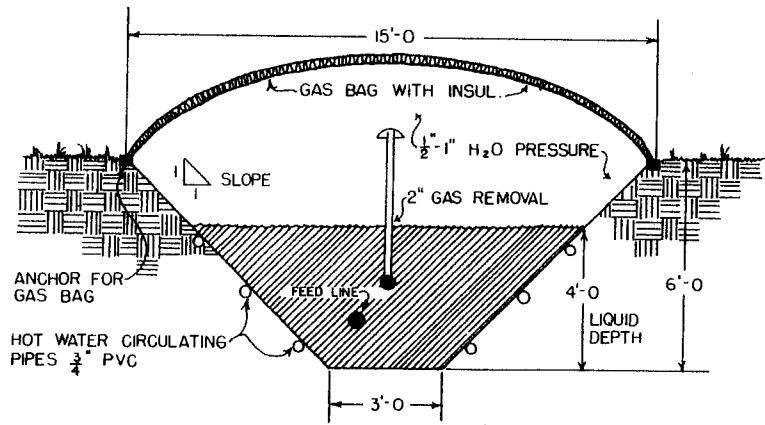
END SECTION SCALE: \frac{3}{8} " = 1'-0"
