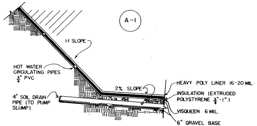
BOTTOM DETAIL SCALE: 1" = 1'-0"
